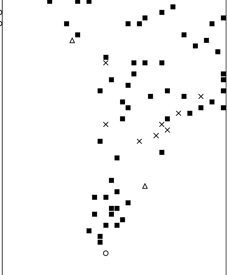
Basisplaat 5 161 = ■ 179 = ○ 250 = × 270 = △
