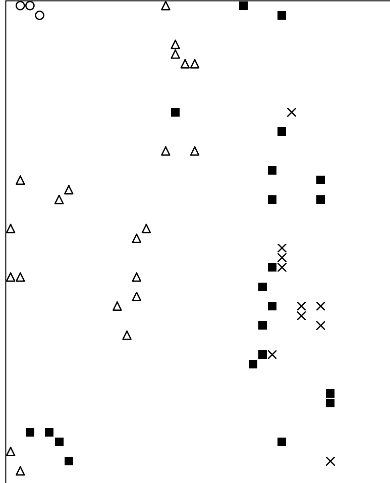
Basisplaat 3 101 = ■ 118 = ○ 120 = × 130 = △
