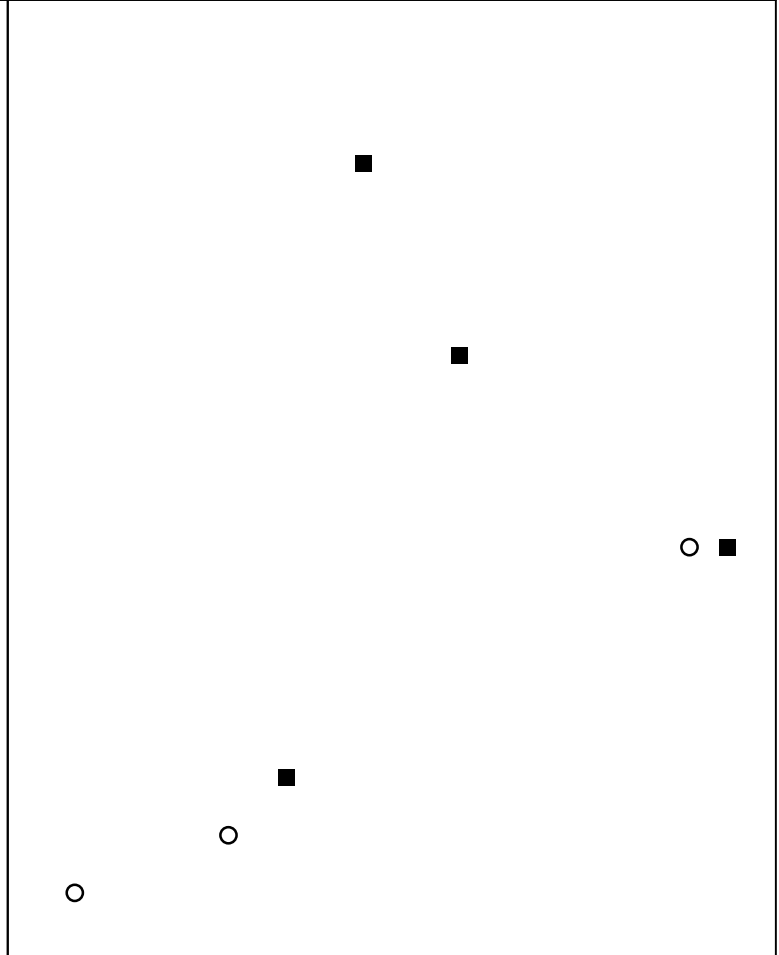
Basisplaat 6 546 = ■ 549 = ○
