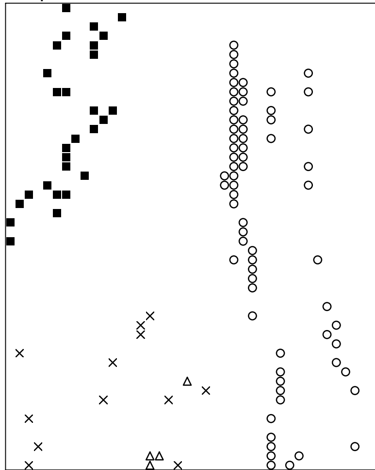
Basisplaat 4 296 = ■ 307 = ○ 319 = × 323 = △
