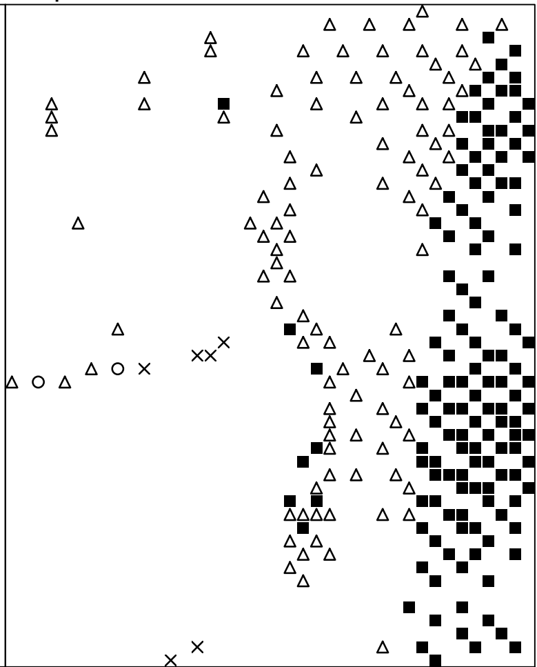
Basisplaat 8 271 = ■ 273 = ○ 283 = × 307 = △
