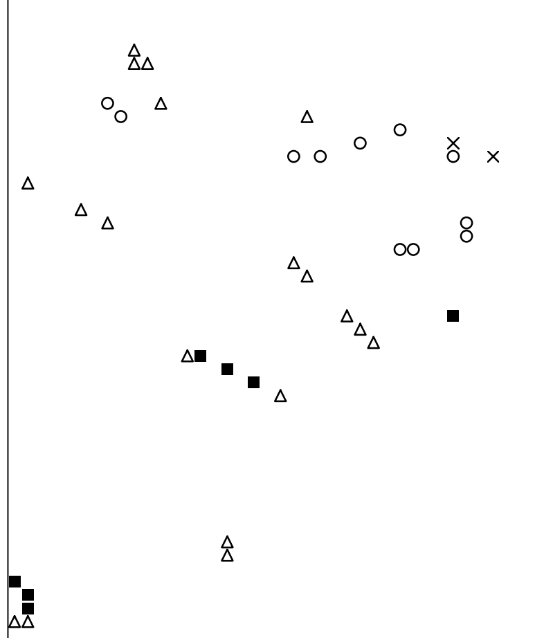
Basisplaat 1 151 = ■ 153 = ○ 158 = × 171 = △
