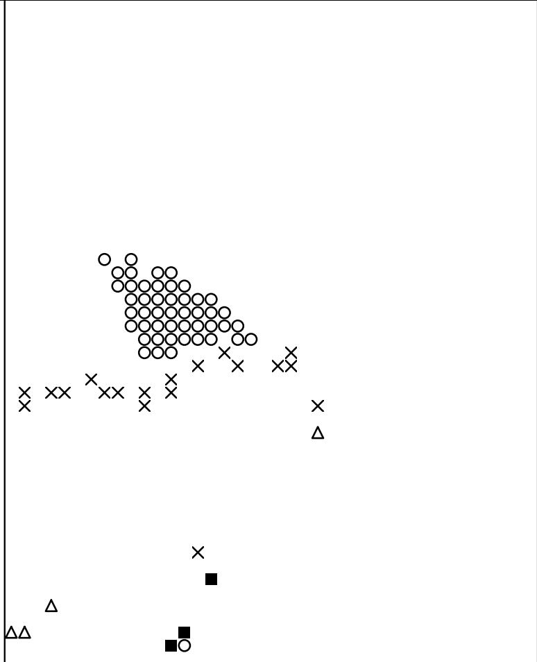
Basisplaat 8 486 = ■ 487 = ○ 513 = × 514 = △
