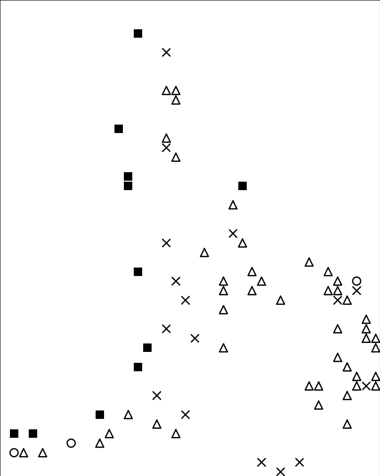
Basisplaat 6 307 = ■ 330 = ○ 339 = × 353 = △
