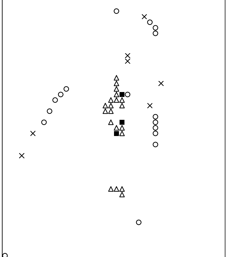
Basisplaat 4 408 = ■ 409 = ○ 411 = × 412 = △
