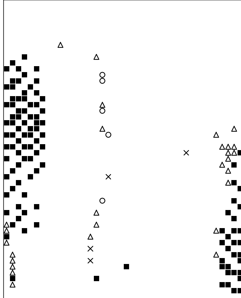
Basisplaat 5 271 = ■ 273 = ○ 274 = × 307 = △
