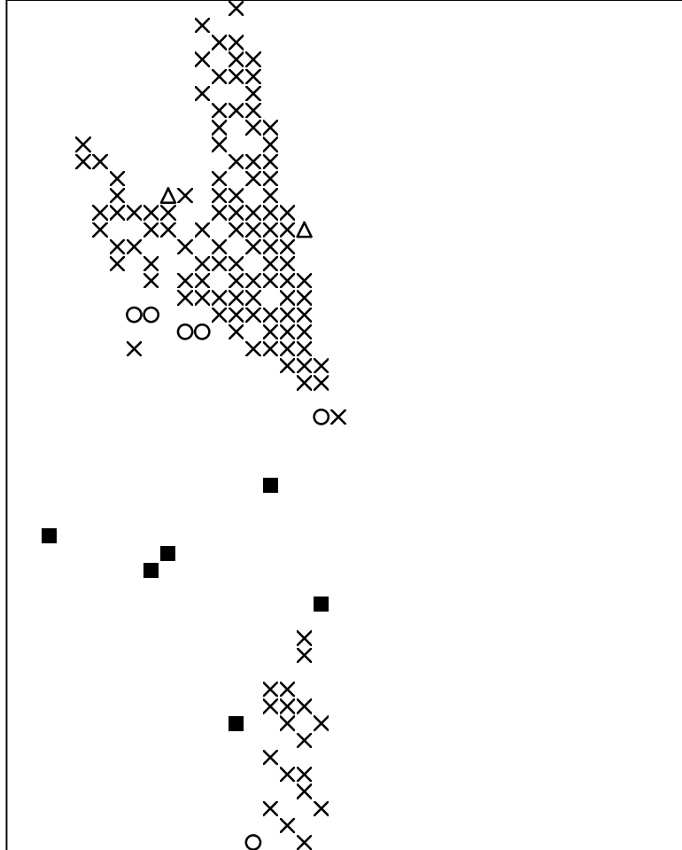
Basisplaat 8 161 = ■ 171 = ○ 172 = × 173 = △
