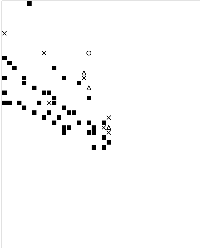
Basisplaat 7 429 = ■ 474 = ○ 479 = × 481 = △
