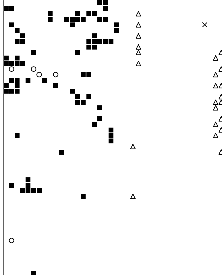
Basisplaat 3 258 = ■ 262 = ○ 270 = × 271 = △
