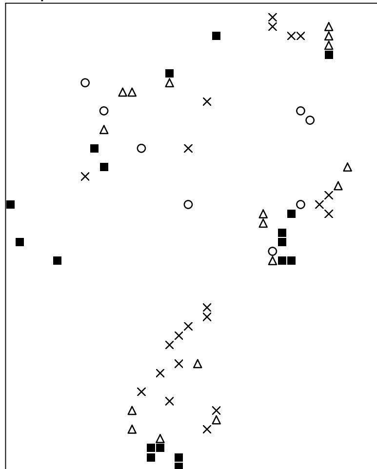
Basisplaat 1 189 = ■ 191 = ○ 193 = × 201 = △
