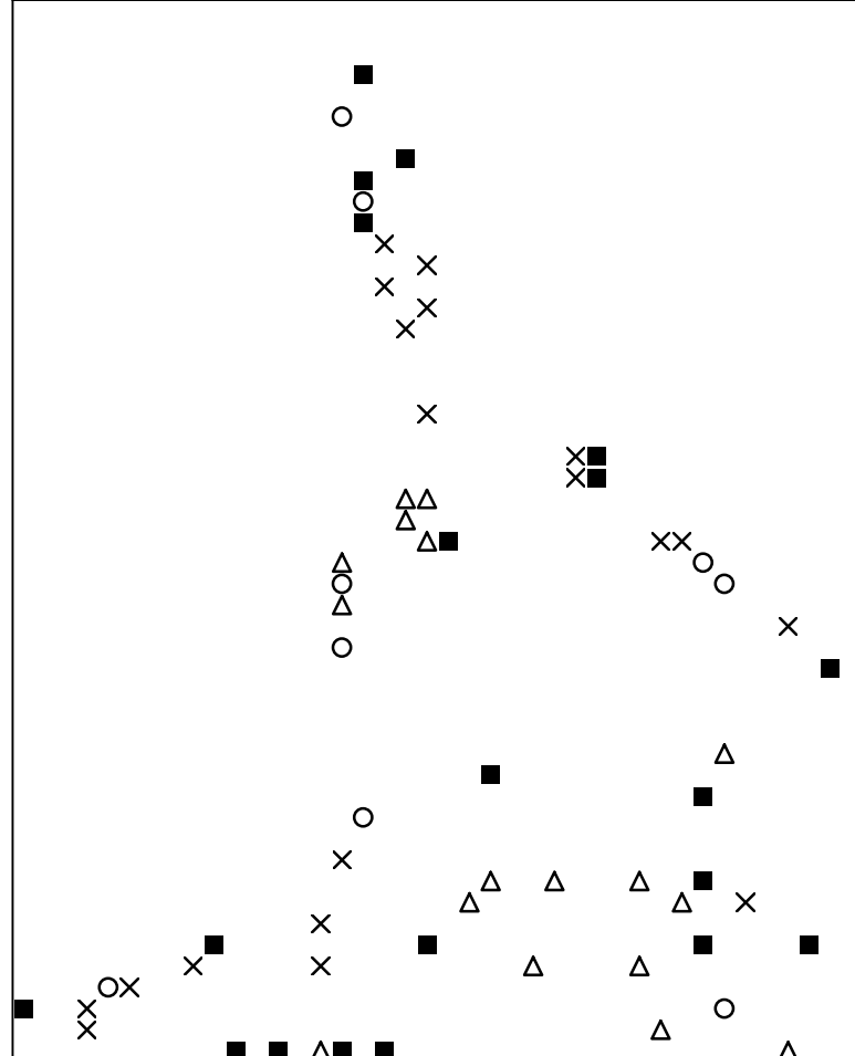
Basisplaat 6 479 = ■ 481 = ○ 513 = × 514 = △
