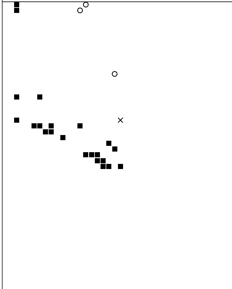
Basisplaat 7 514 = ■ 546 = ○ 549 = ×
