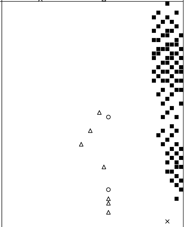
Basisplaat 4 271 = ■ 273 = ○ 274 = × 283 = △
