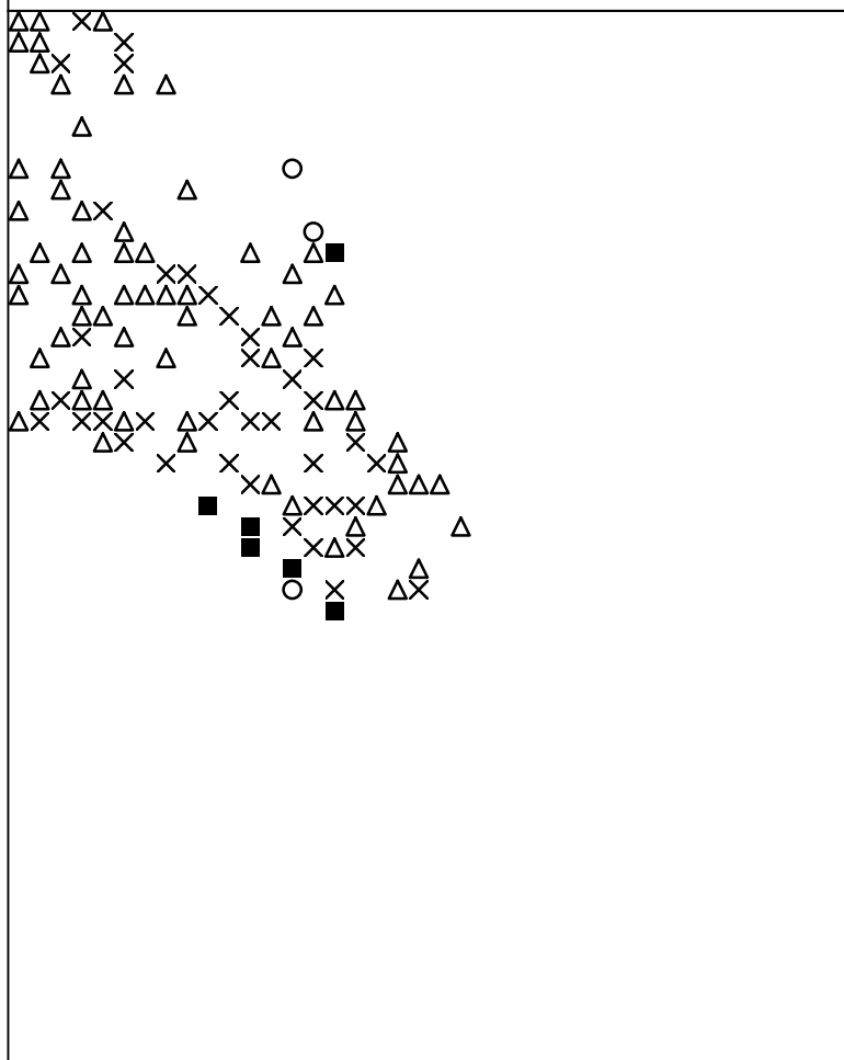
Basisplaat 7 371 = ■ 376 = ○ 389 = × 394 = △
