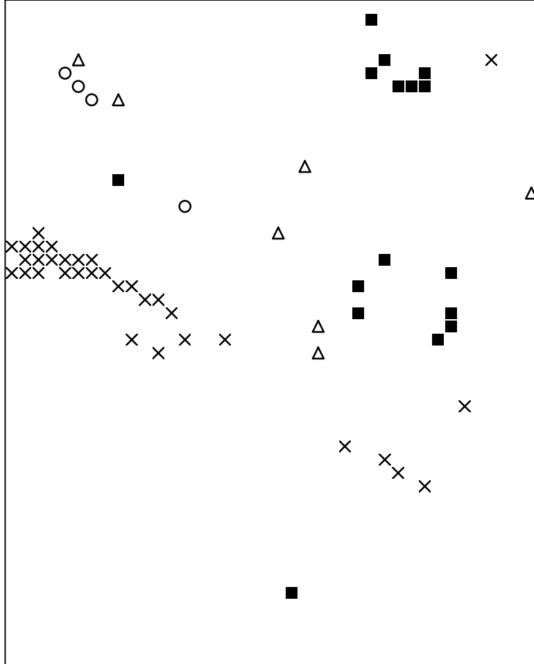
Basisplaat 1 469 = ■ 474 = ○ 483 = × 484 = △
