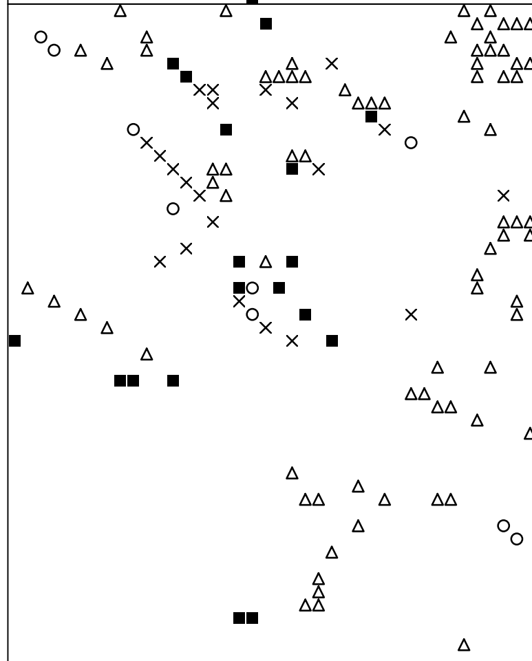
Basisplaat 1 227 = ■ 233 = ○ 236 = × 258 = △
