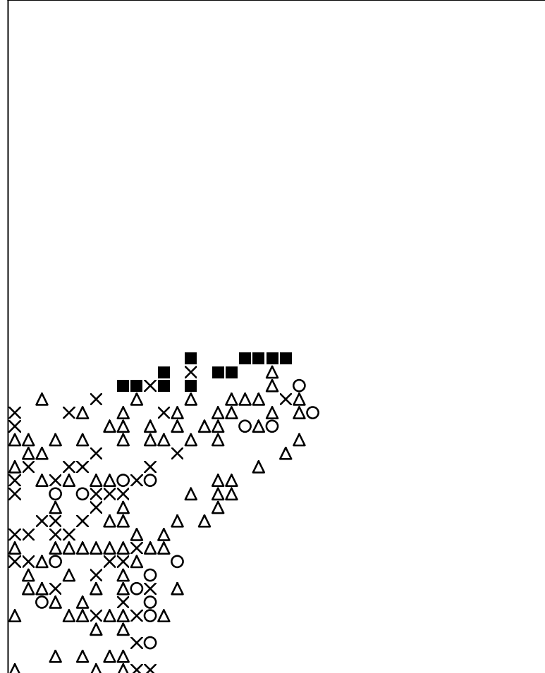
Basisplaat 8 330 = ■ 339 = ○ 353 = × 354 = △
