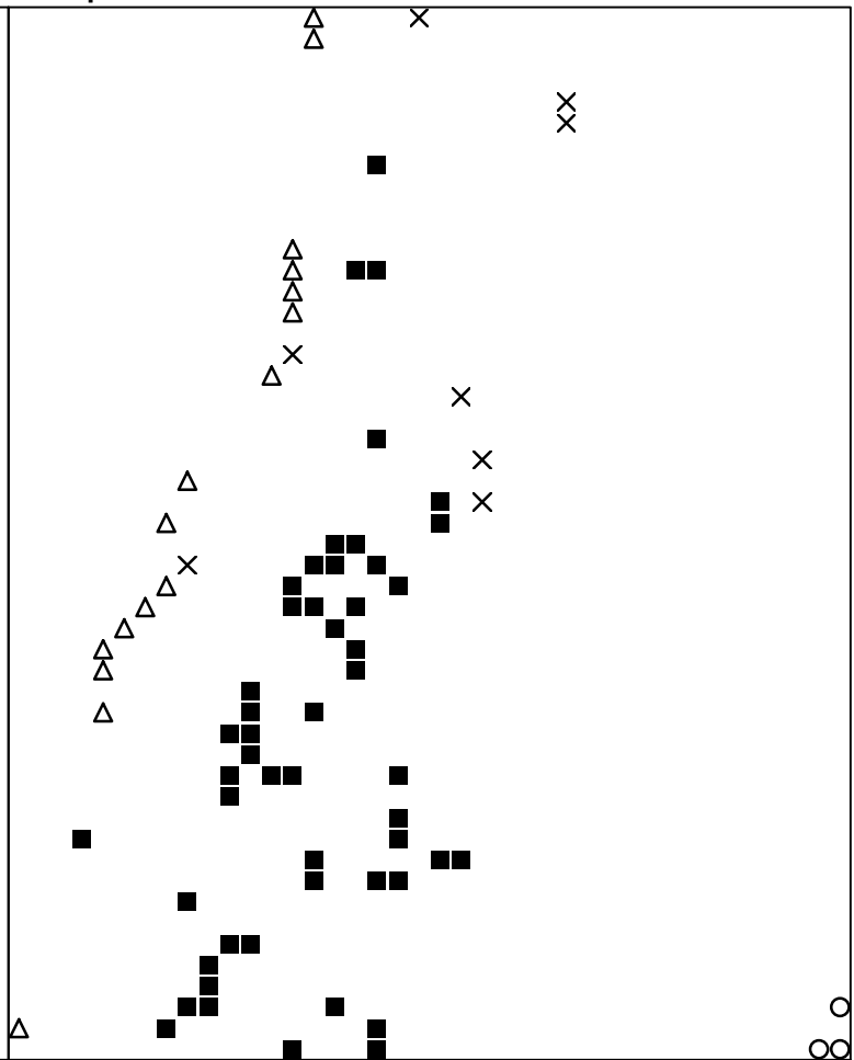
Basisplaat 4 330 = ■ 354 = ○ 358 = × 359 = △
