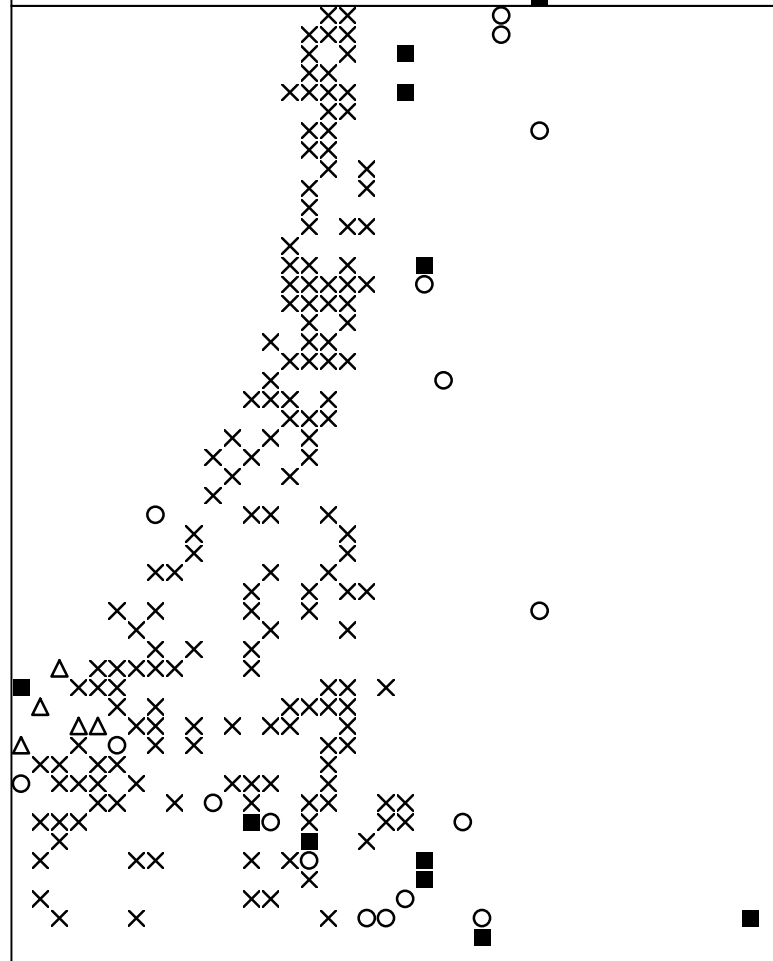
Basisplaat 4 233 = ■ 236 = ○ 258 = × 262 = △
