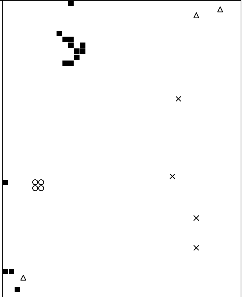
Basisplaat 3 131 = ■ 133 = ○ 141 = × 158 = △
