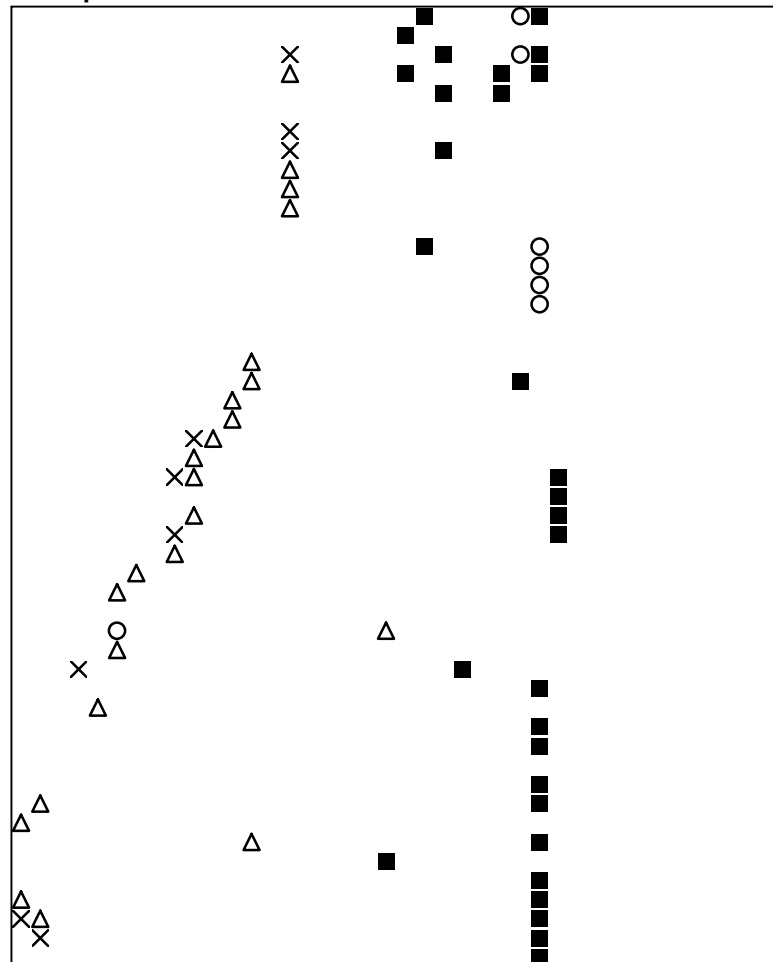
Basisplaat 4 191 = ■ 193 = ○ 201 = × 211 = △
