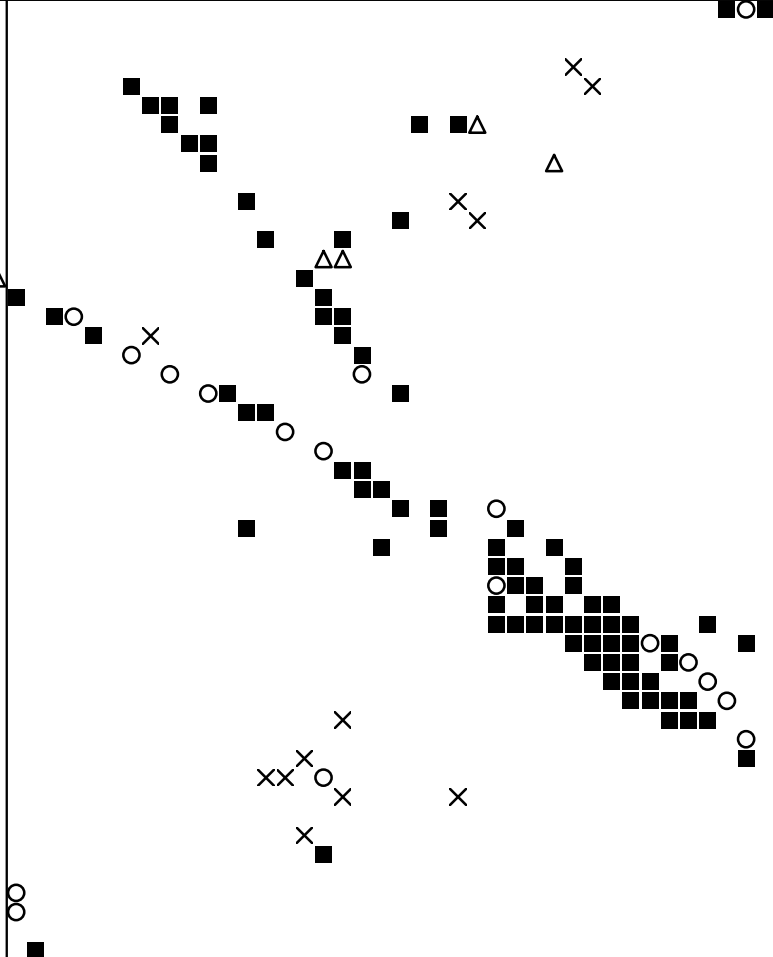
Basisplaat 1 486 = ■ 487 = ○ 494 = × 513 = △
