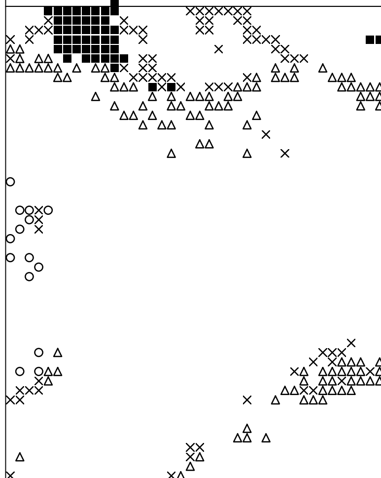
Basisplaat 2 341 = ■ 358 = ○ 364 = × 365 = △
