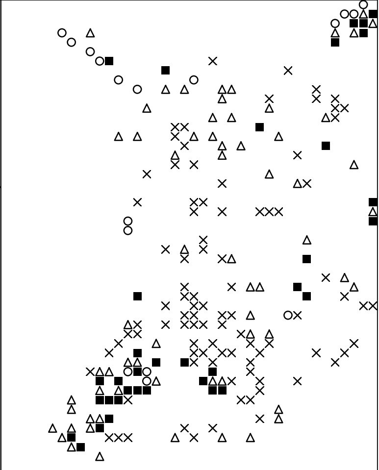
Basisplaat 1 547 = ■ 548 = ○ 549 = × 550 = △
