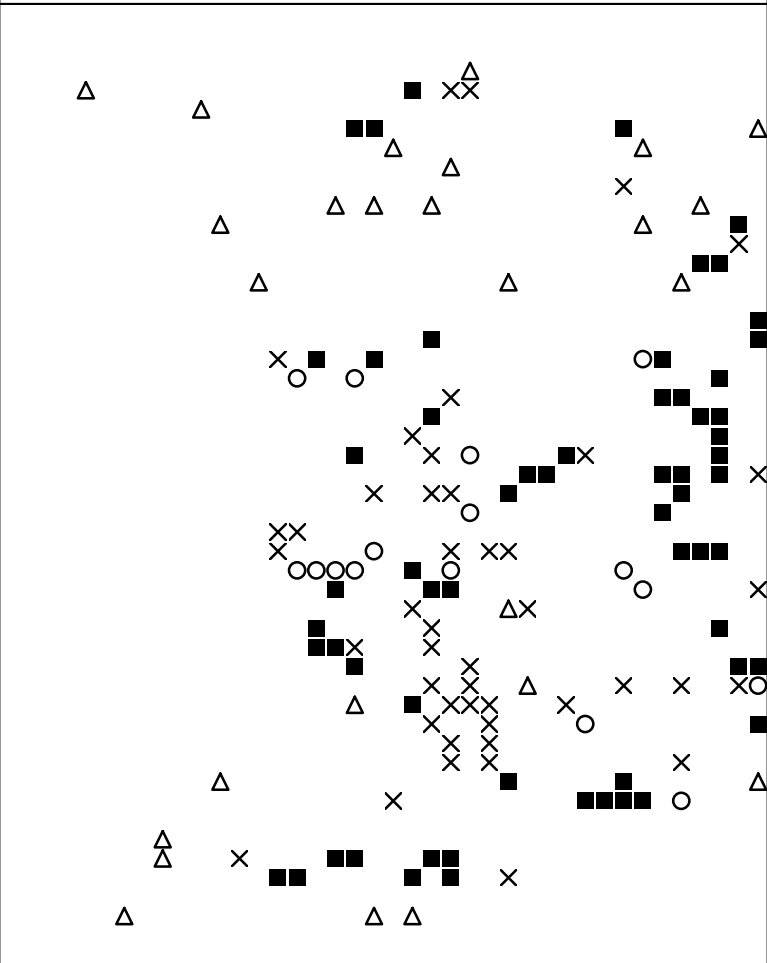
Basisplaat 1 317 = ■ 323 = ○ 325 = × 327 = △
