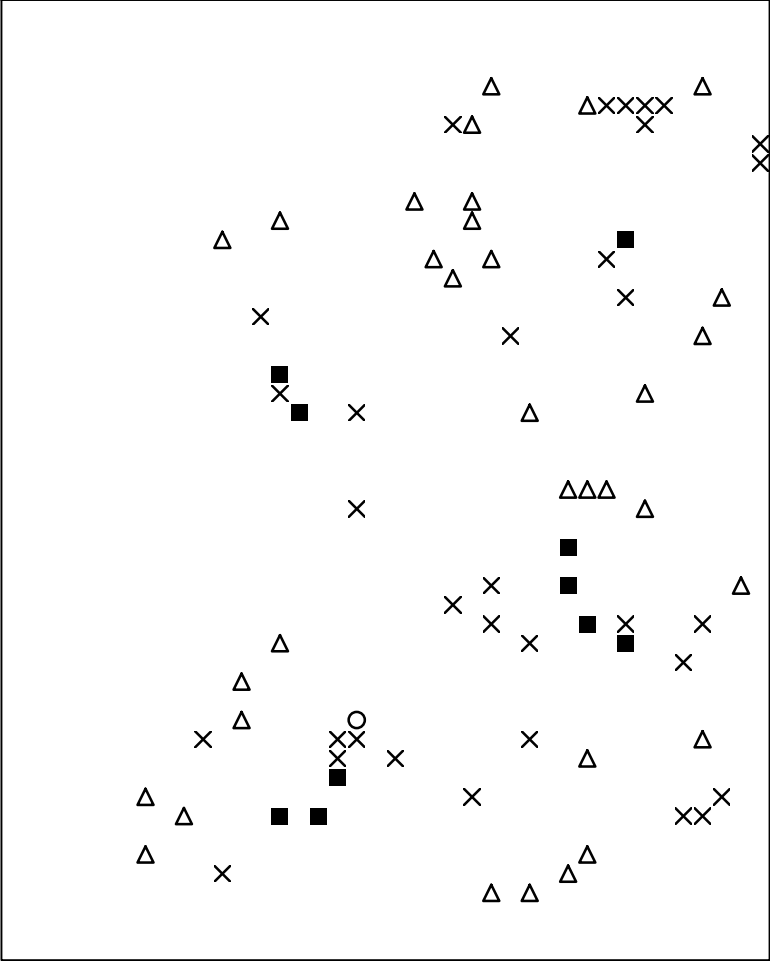
Basisplaat 1 183 = ■ 191 = ○ 227 = × 228 = △
