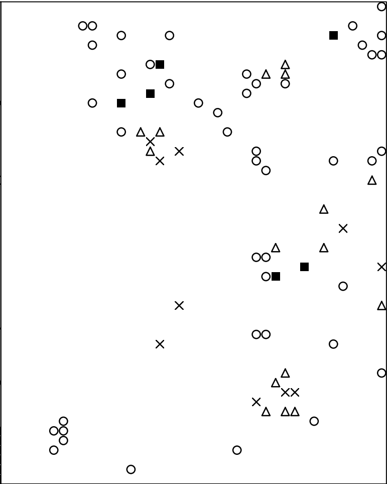
Basisplaat 1 173 = ■ 175 = ○ 178 = × 179 = △
