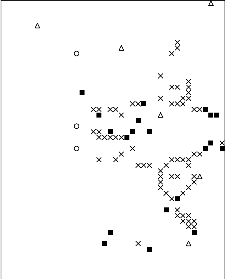
Basisplaat 1 393 = ■ 411 = ○ 412 = × 414 = △
