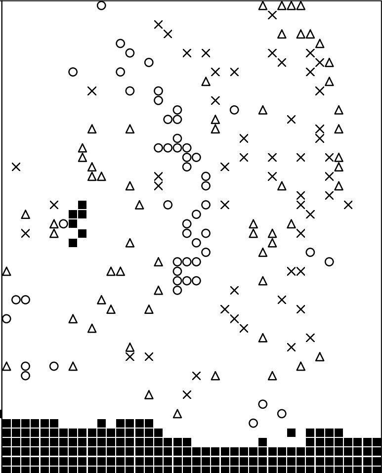
Basisplaat 2 100 = ■ 101 = ○ 104 = × 170 = △
