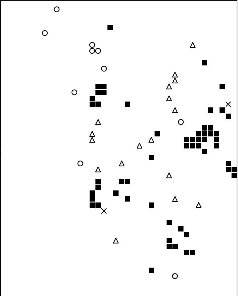
Basisplaat 1 461 = ■ 474 = ○ 481 = × 483 = △
