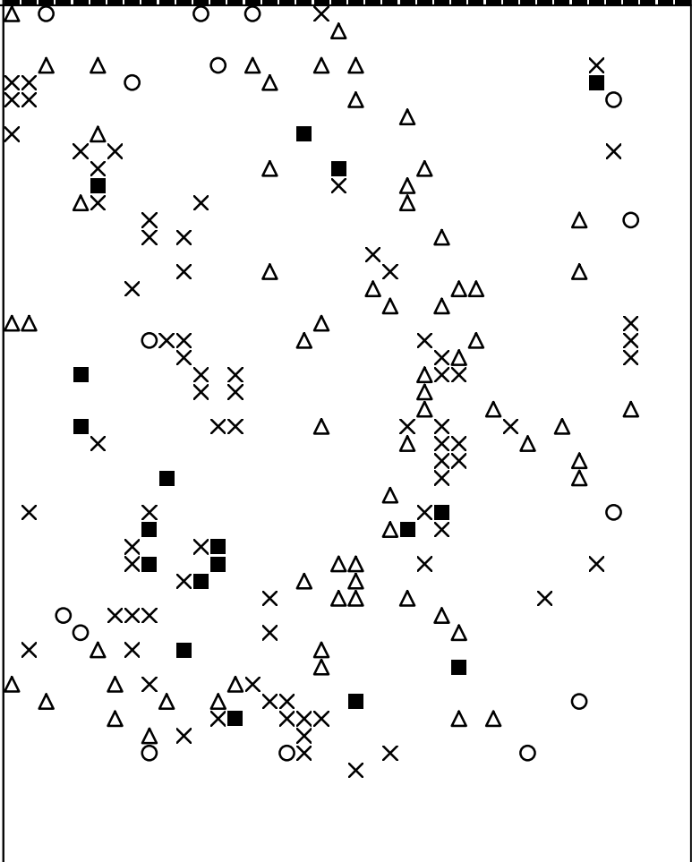
Basisplaat 2 183 = ■ 191 = ○ 227 = × 228 = △
