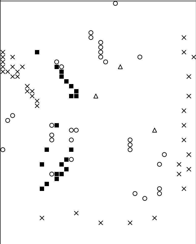
Basisplaat 2 283 = ■ 297 = ○ 307 = × 310 = △
