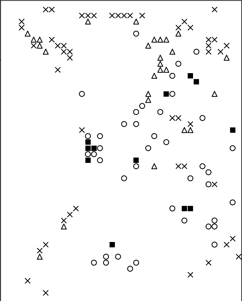
Basisplaat 1 283 = ■ 297 = ○ 307 = × 310 = △
