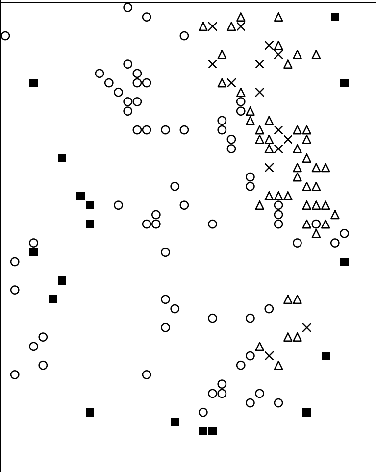
Basisplaat 2 173 = ■ 175 = ○ 178 = × 179 = △
