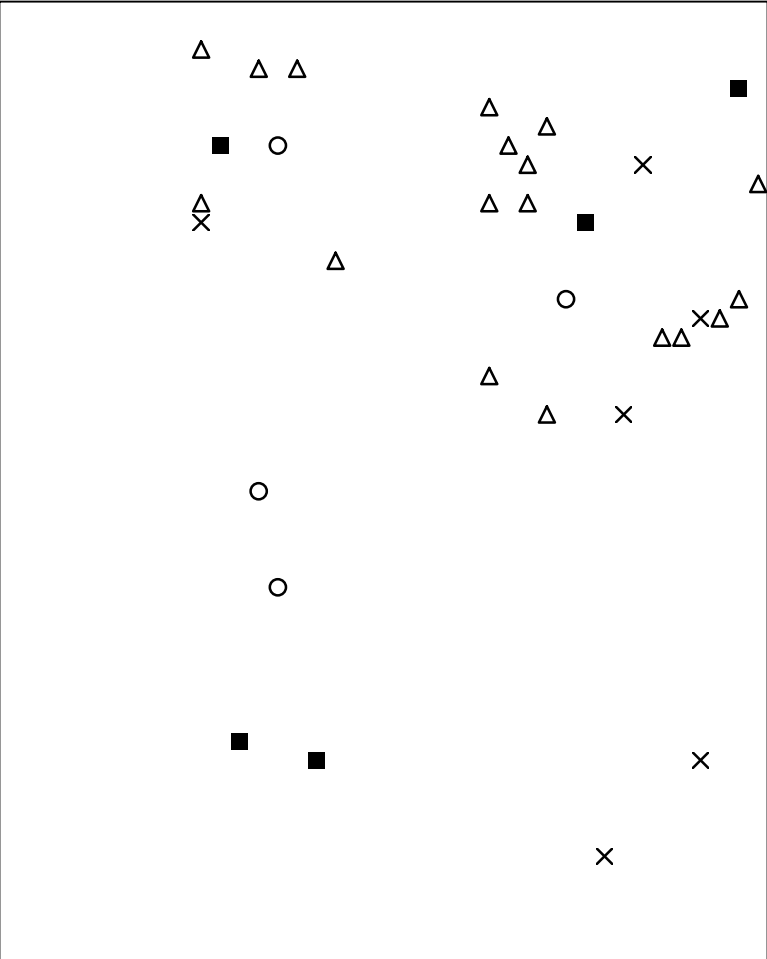
Basisplaat 1 236 = ■ 237 = ○ 264 = × 274 = △
