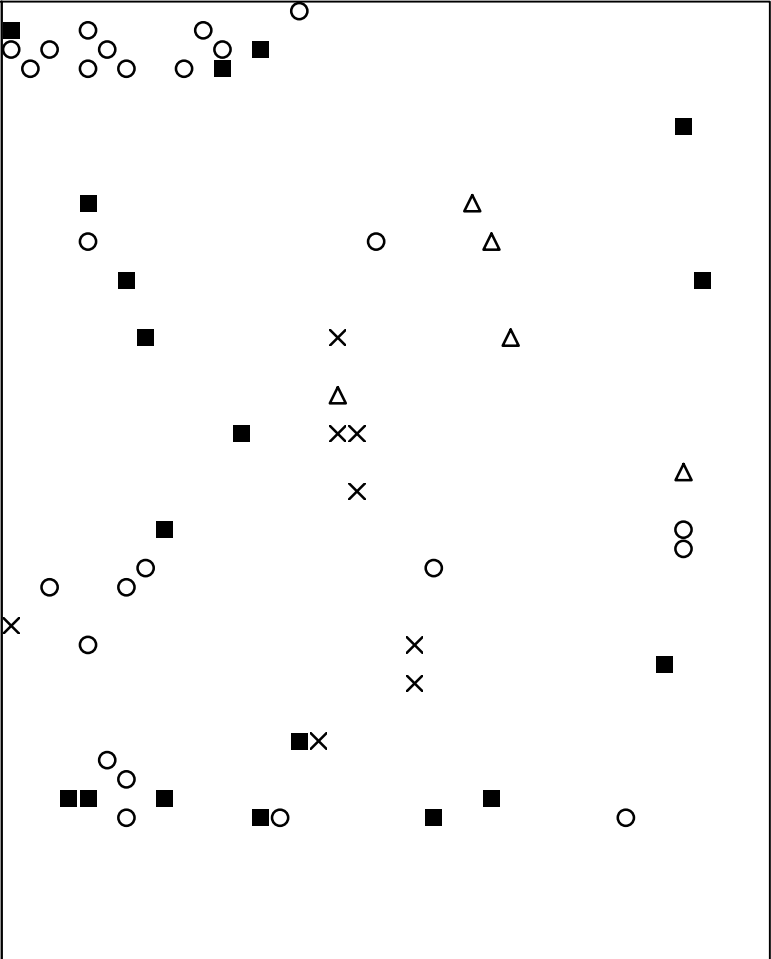
Basisplaat 2 236 = ■ 237 = ○ 264 = × 274 = △
