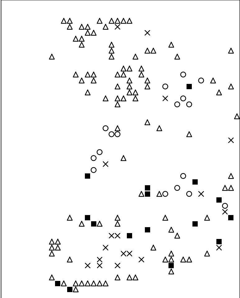
Basisplaat 1 484 = ■ 486 = ○ 489 = × 546 = △
