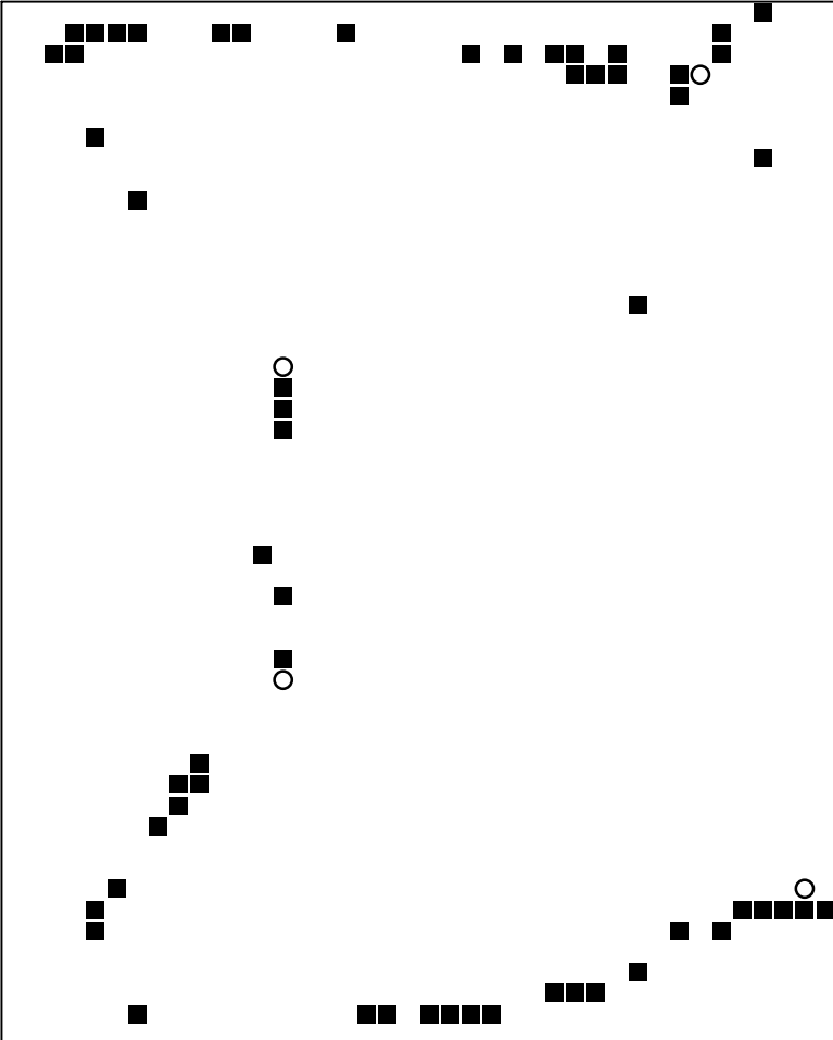
Basisplaat 1 552 = ■ 553 = ○
