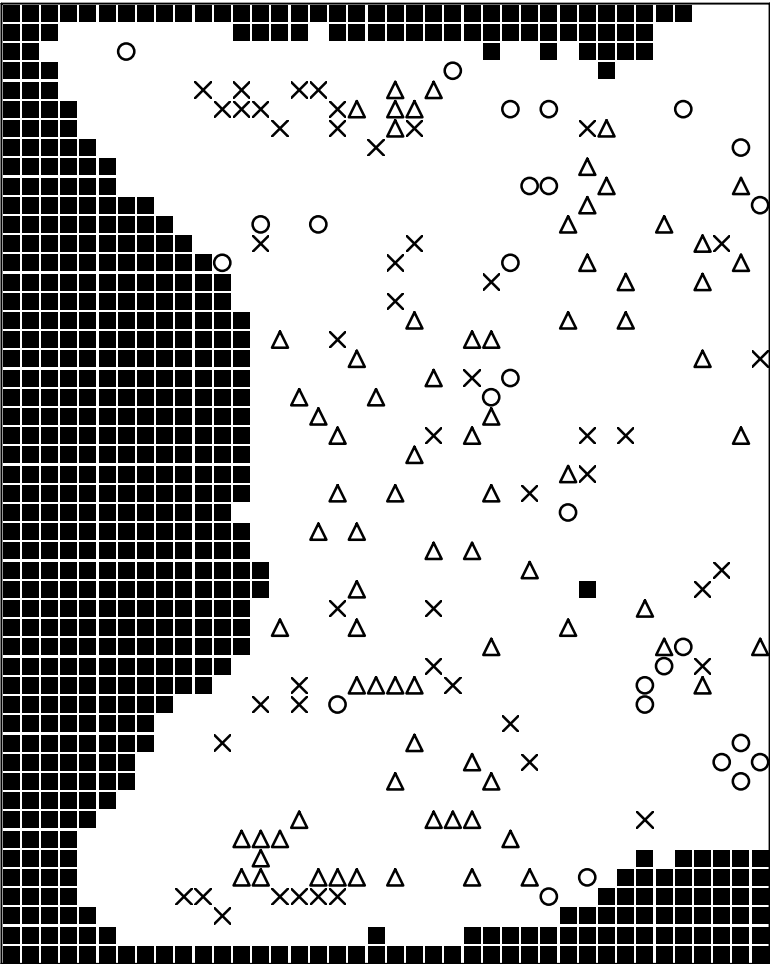
Basisplaat 1 100 = ■ 101 = ○ 104 = × 170 = △
