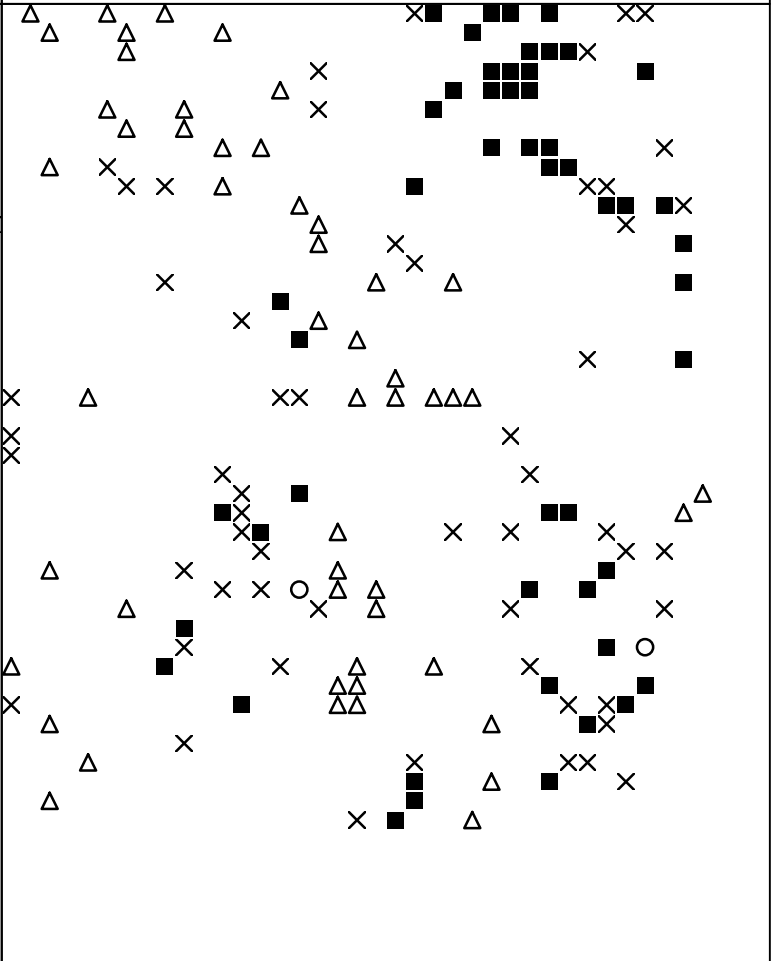
Basisplaat 2 317 = ■ 323 = ○ 325 = × 327 = △
