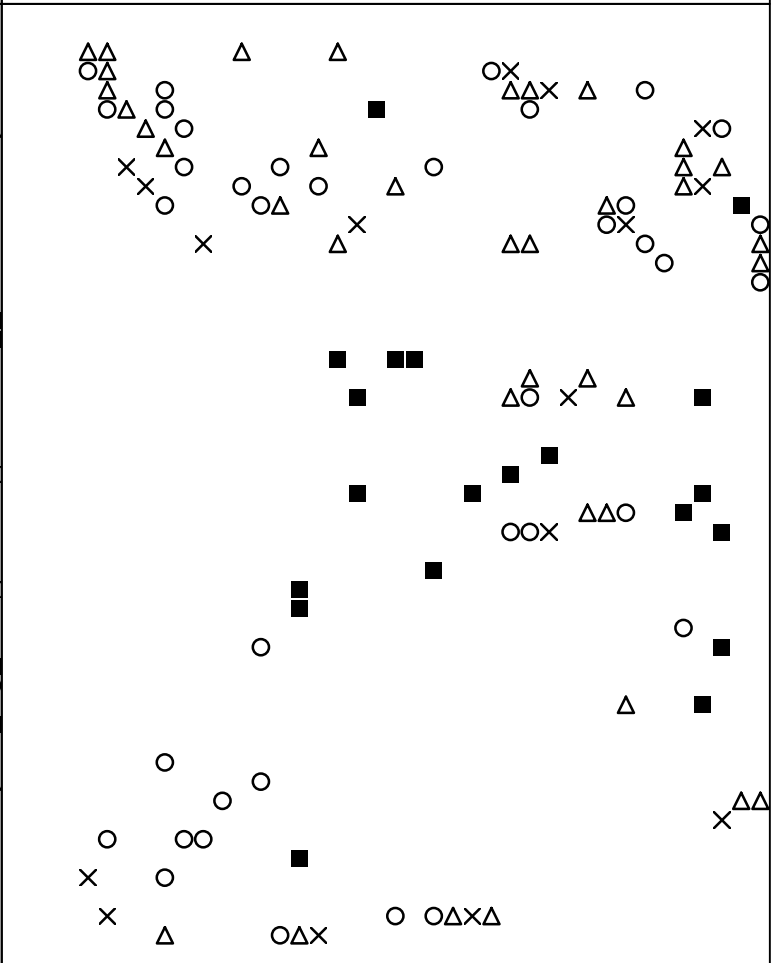
Basisplaat 1 330 = ■ 374 = ○ 375 = × 388 = △
