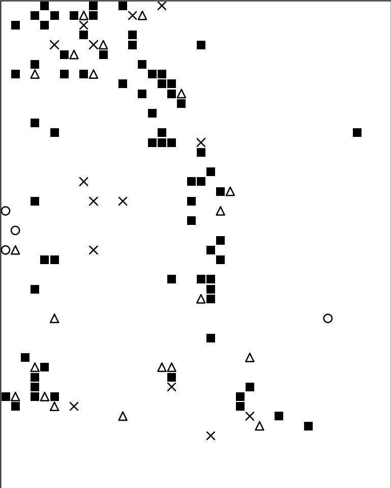
Basisplaat 2 229 = ■ 230 = ○ 231 = × 233 = △
