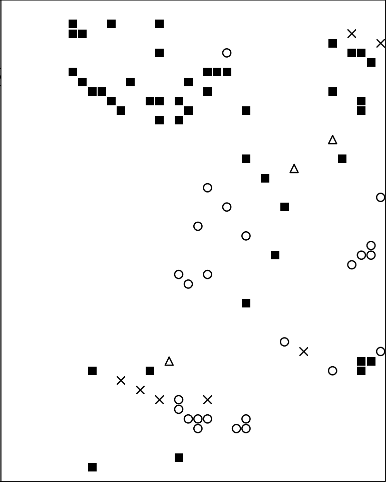
Basisplaat 1 229 = ■ 230 = ○ 231 = × 233 = △
