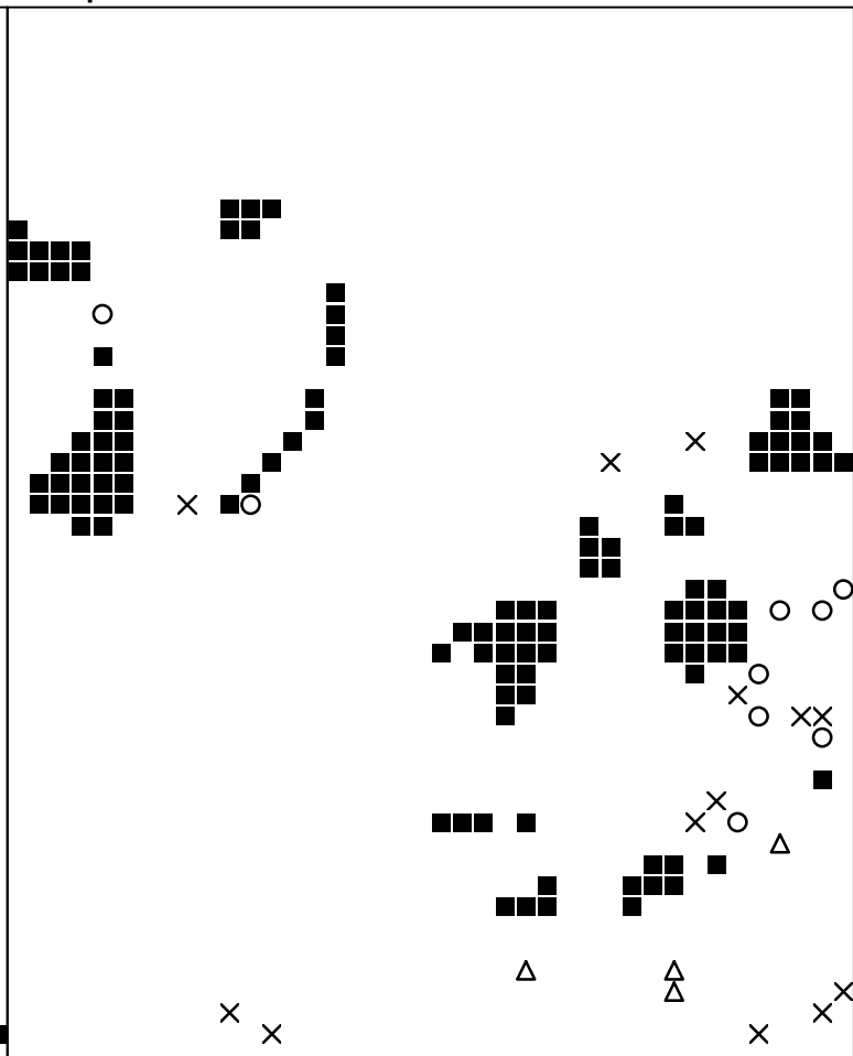
Basisplaat 7 100 = ■ 101 = ○ 108 = × 115 = △
