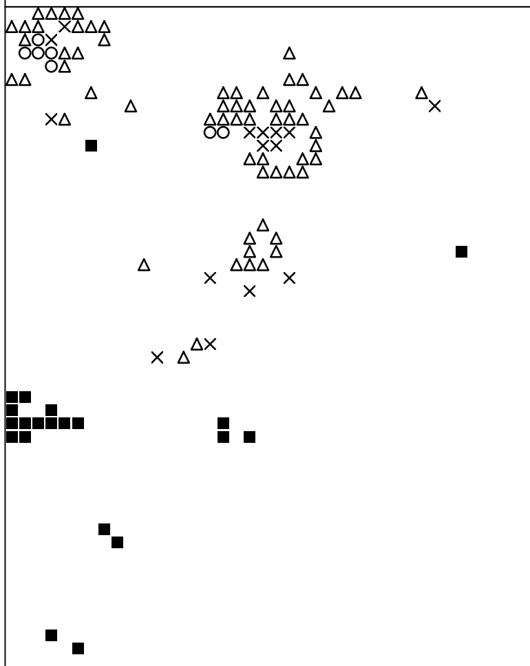
Basisplaat 7 117 = ■ 126 = ○ 130 = × 131 = △
